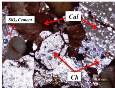
شکل ۴. مقاطع نازک میکروسکوپی و نتایج آنالیزهای XRD تعدادی از نمونه‌های مورد مطالعه الف) ژئیس ب) کنگلومرا
