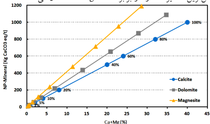
شکل ۶. ارتباط بین NP کانی‌شناسی با غلظت Ca+Mg برای گونه‌های کربناتی مختلف
