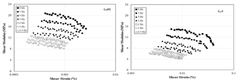
شکل ۱۳. تغییرات مدول برشی با کرنش برشی در فرکانس‌های مختلف بارگذاری تحت بارگذاری مثالی و شتاب ورودی الف) 0.1g ، ب) 0.3g
