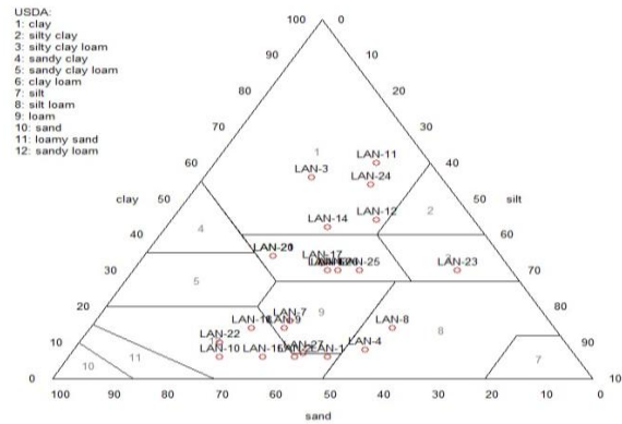
شکل ۳. نمودار مثلثی بافت خاک‌های محل دفن زباله
