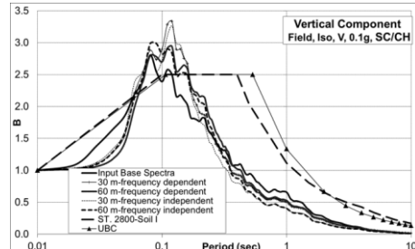
ب) موج برشی صحرایی، مینا سرعت PGA=0.1g ، خاک نوع I، مینا سرعت موج
