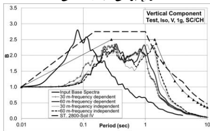
ه) موج برشی آزمایشگاهی، مینا سرعت PGA=1g ، خاک نوع IV، مینا سرعت موج
