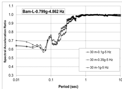
الف) زلزله بم با فرکانس غالب 4/9 Hz
