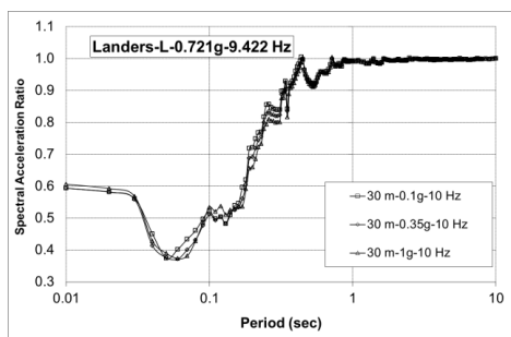
ب) زلزله لندرز (رکورد LCN) با فرکانس غالب
