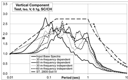
الف) موج برشی آزمایشگاهی، مینا سرعت PGA=0.1g ، خاک نوع IV، مینا سرعت
