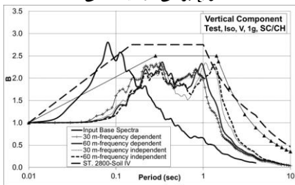
ه) موج برشی آزمایشگاهی، خاک نوع IV، مینا سرعت PGA=1g
