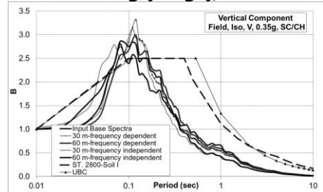
د) موج برشی صحرایی، خاک نوع I، مینا سرعت PGA=0.35g
