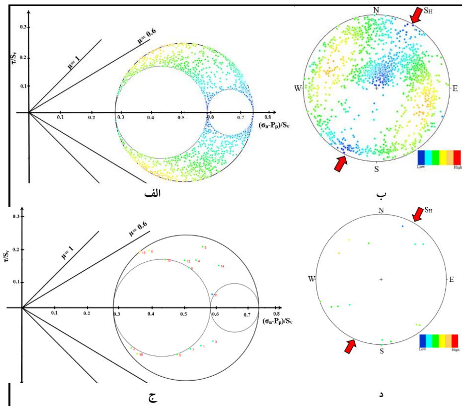
شکل ۱۵. الف و ب) وضعیت شکستگی‌ها بعد از برداشت و افت فشار در مخزن به میزان 8/76 مگاپاسگال، ج و د) وضعیت گسل‌ها بعد از برداشت و افت فشار در مخزن را نشان می‌دهند (رنگ‌های گرم نشان‌دهنده پتانسیل زیاد برای فعالیت و رنگ‌های سرد نشان‌دهنده پتانسیل کم برای فعالیت است).
