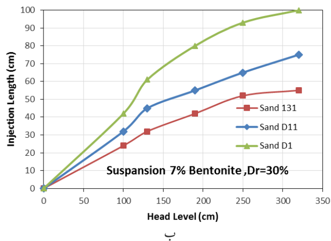
شکل ۵. تغییرات طول نفوذ در برابر تراز فشار تزریق برای نمونه با درصد تراکم ۳۰٪ و غلظت دوغاب برابر الف (۵٪، ب) ۷٪ بنتونیت در ماسه‌های مختلف
