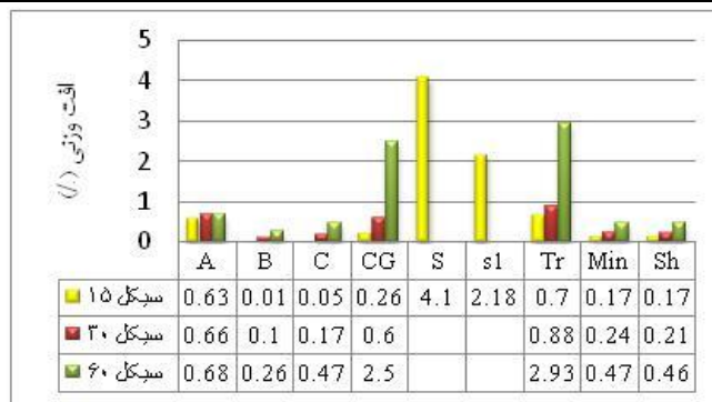
شکل ۳. تغییر خصوصیات فیزیکی و مکانیکی ماسه سنگ‌های بررسی شده با سیکل‌های پدیده ذوب-انجماد: الف) درصد افت وزنی،
