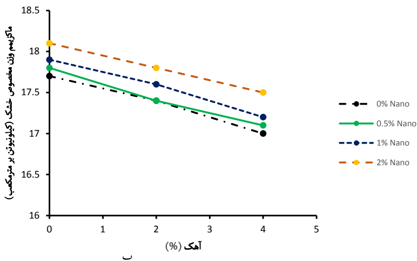
شکل ۱. الف) تأثیر نانو مواد و آهک بر درصد رطوبت بهینه، ب) تأثیر نانو مواد و آهک بر وزن مخصوص خشک بهینه
