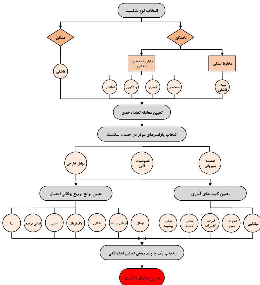
شکل ۳. روند کلی تحلیل احتمالاتی شيرواني‌ها
