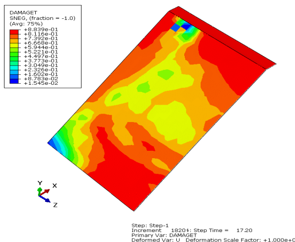
شکل ۱۰. مقایسه خرابی روکش بتنی تحت زلزله طیس در سه حالت؛ الف) خالی، ب) نیمه پر و ج) پر
