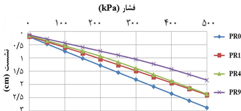
شکل ۳. منحنی‌های بار-نشست دال در حالت شمع‌های متصل (نماد PR به معنای شمع متصل و اعداد بعد از آن نشان‌دهنده تعداد شمع است)
