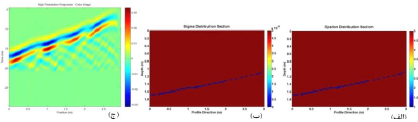
شکل ۵. الف) مقطع توزیع گذردهی دی‌الکتریک، ب) مقطع توزیع هدایت الکتریکی و ج) پاسخ GPR مدل منشور دوبعدی گرانیتی شامل یک ناپوستگی سرتاسری
