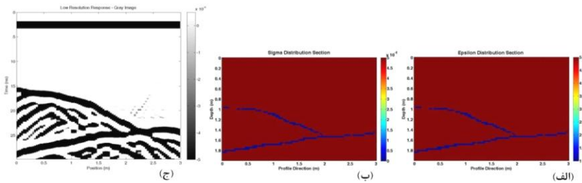
شکل ۶. الف) مقطع توزیع گذردهی دی‌الکتریک، ب) مقطع توزیع هدایت الکتریکی و ج) پاسخ GPR مدل منشور دوبعدی گرانیتی شامل دو ناپوستگی متقاطع
