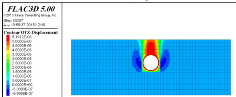
شکل ۱۲. مکانیزم گسیختگی خاک طی برخواست لوله در خاک غیرمسلح
