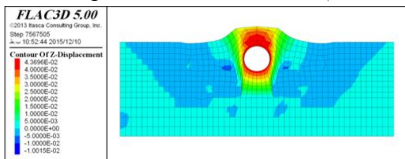
شکل ۱۴. مکانیزم گسیختگی خاک طی برخواست لوله در خاک مسلح با سیستم مهار- شبکه
