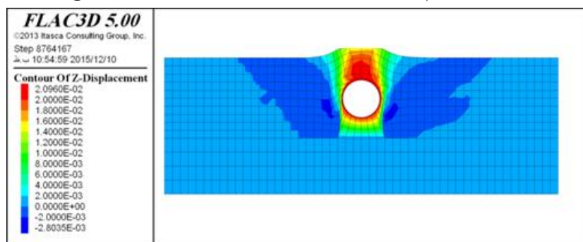
شکل ۱۳. مکانیزم گسیختگی خاک طی برخواست لوله در خاک مسلح با ژئوگرید تنها
