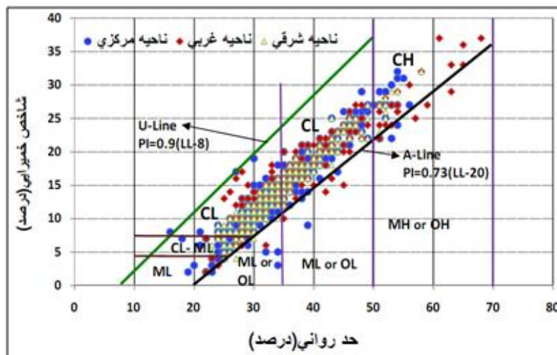
شکل ۵. نمودار پلاستیسیته نهشته‌های زیربهنه شهر کرمان مربوط به نواحی سه‌گانه
