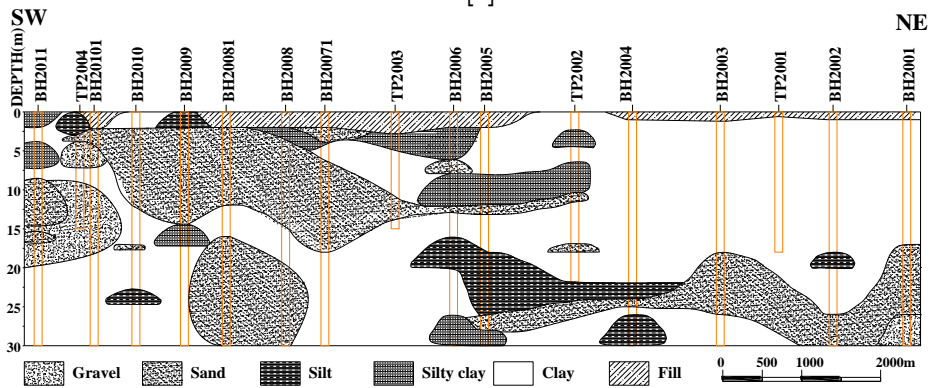
شکل ۲. مقطع زمین‌شناسی مسیر خط ۲ قطار شهری مشهد به همراه جانمایی گمانه‌ها
