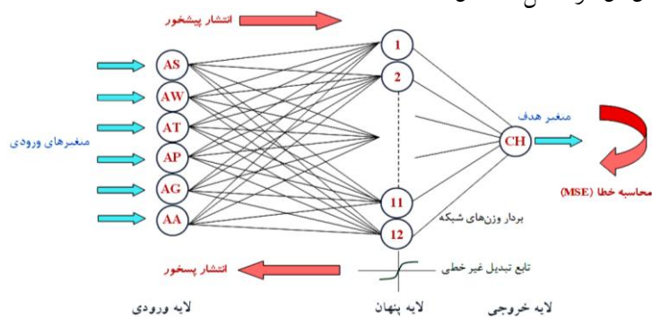
شکل ۴. معماری شبکه
