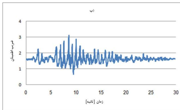
شکل ۵. تاریخچه زمانی ضریب اطمینان گوه مستعد لغزش در حالت تحریک با زلزله طیس (الف) قبل از اعمال فیلتر بالاگذر
