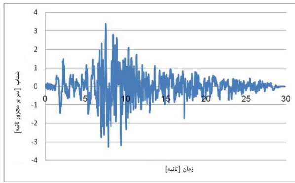
شکل ۳. شتاب‌نگاشت مقیاس شده زلزله طیس
