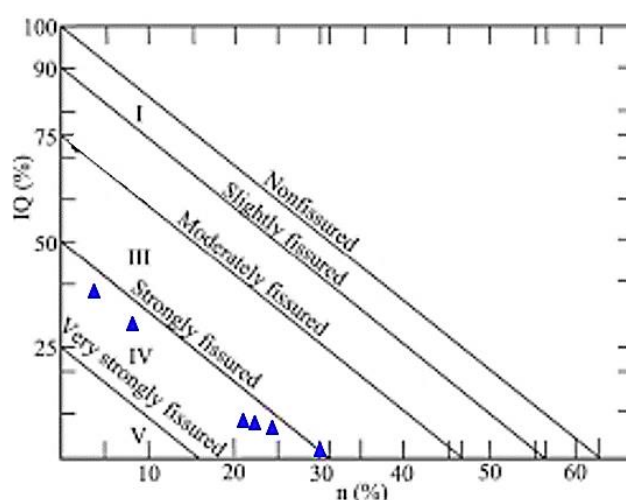
شکل ۱۰. موقعیت نمونه ها در رده بندی شاخص ترک خوردگی (Fourmaintraux, 1976)
