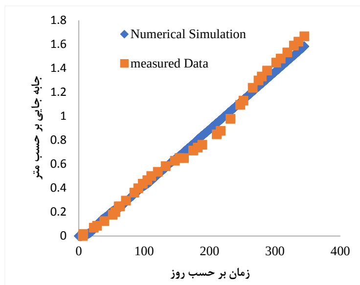
شکل ۵. مقایسه جابه‌جایی‌های محاسبه شده توسط مدل عددی و اندازه‌گیری‌های برجای برای نقطه شاهد ۱۳۶۰-۰۵۱ Fig. 5. Comparison of displacements calculated by the numerical model and in-situ measurements for reference point 051-1360
