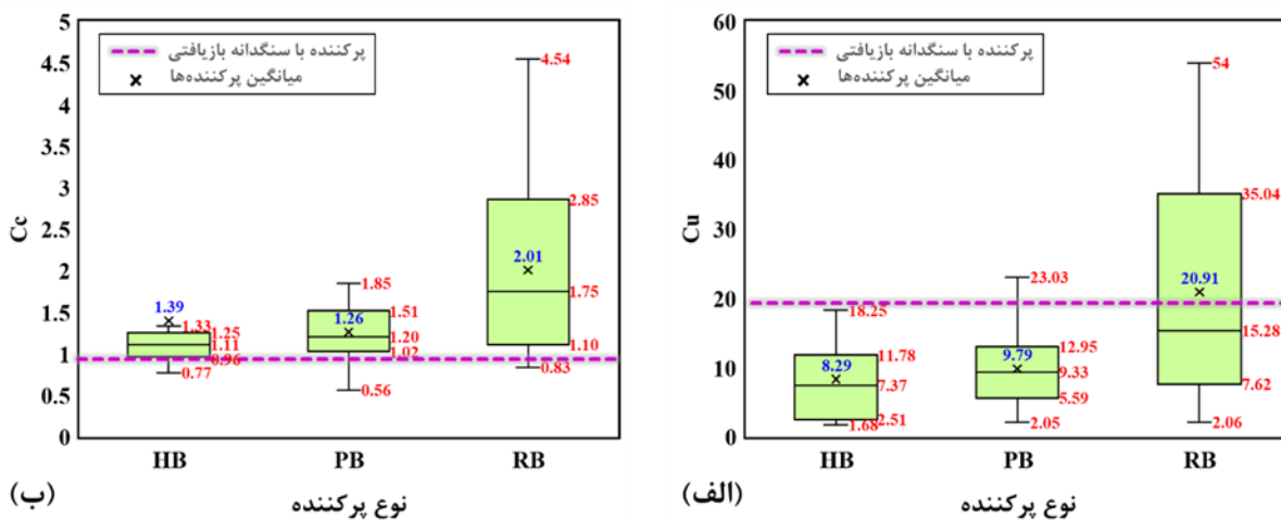
شکل ۲۰. نمودار جعبه‌ای مربوط به (الف) ضریب یکنواختی و (ب) ضریب انحنای پرکننده‌های هیدرولیکی، خمیری و سنگی به همراه پرکننده حاصل از سنگدانه بازیافتی
