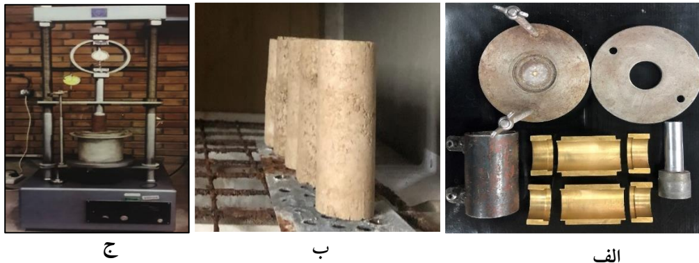
شکل ۱- الف) اجزای قالب مورد استفاده برای ساخت نمونه‌های آزمایشی، ب) نحوه نگهداری نمونه‌ها در اتاقک مخصوص و ج) دستگاه بارگذاری تک‌محوری مورد استفاده
