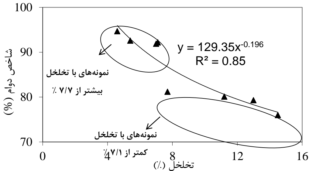
شکل ۱۱. رابطه دوام نمونه‌ها در آزمایش دوام و ارتنگی در محلول اشباع نمک و تخلخل
