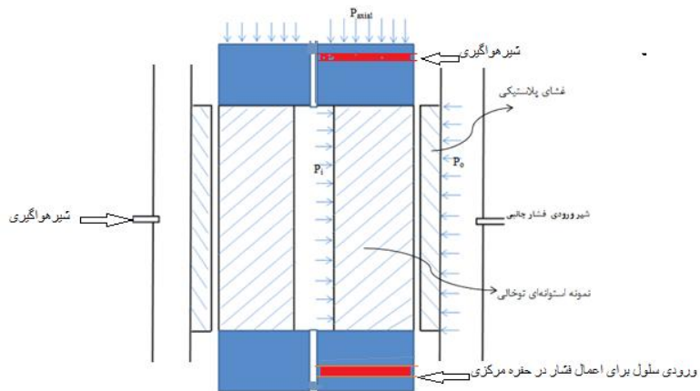
شکل ۳. نمایی از طراحی انجام شده برای اعمال فشار داخلی در سلول هوک تغییر یافته (در شکل نشان‌دهنده تنش محوری، P_{axial} نشان‌دهنده تنش جانبی و P_0 نشان‌دهنده فشار در حفره مرکزی است)
