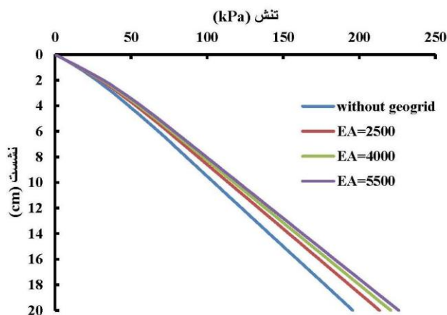
شکل ۸. نمودار تنش - نشست با ژئوگرید به طول 0.5L و برای سختی های متفاوت در شرایطی که S=2\text{ m}
