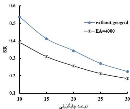
شکل ۱۵. تأثیر درصد جایگزینی روی نسبت نشست
