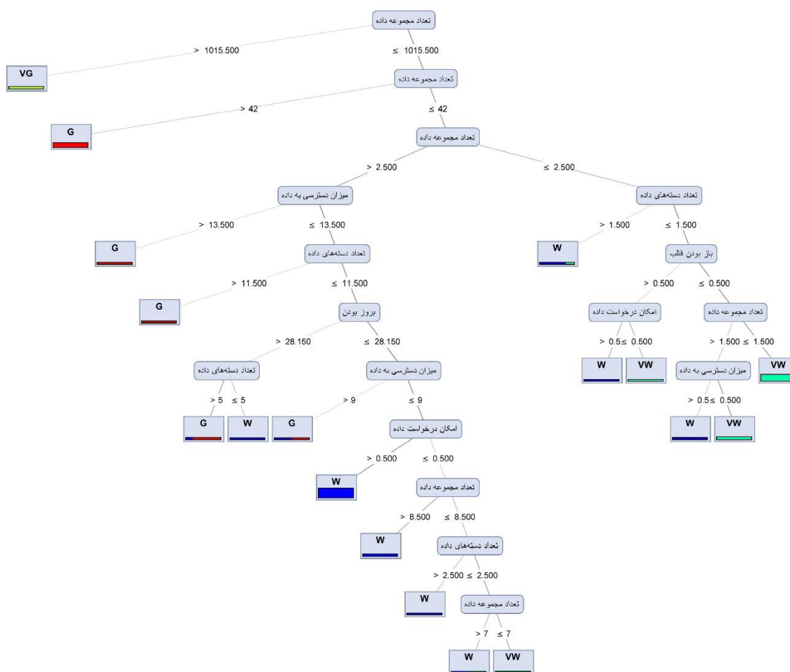
شکل ۱۸. درخت تصمیم
