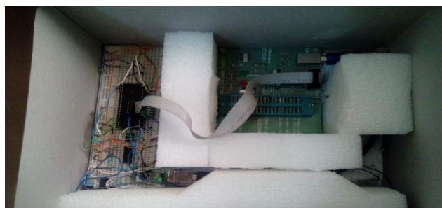
شکل ۱- قسمت الکترونیکی دستگاه تعیین غلظت DNA.
