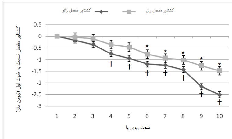
شکل ۳. منحنی نزولی گشتاور مفاصل ران و زانو در طول ۱۰ شوت متوالی روی پا. (* نشان دهنده کاهش معنی دار نسبت به شوت اول در گشتاور مفصل ران و (†) نشان دهنده کاهش معنی دار نسبت به شوت اول در گشتاور مفصل زانو است.
