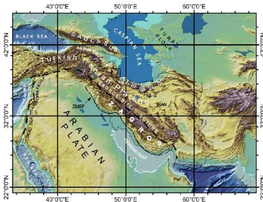
شکل ۱. نقشهٔ کمربند آلپ-همیالیا و موقعیت رشته کوه البرز- تالش در این کمربند برگرفته از جویست ۱ و همکاران (۲۰۰۶) منطقهٔ پژوهش در تالش با مربع مشخص شده است
