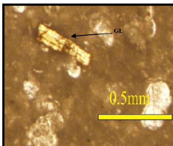
شکل ۱۳. حضور گلوکونیت (GL)، شاهدی از پیش‌روی آب در سکانش چهارم از نمونه G24
