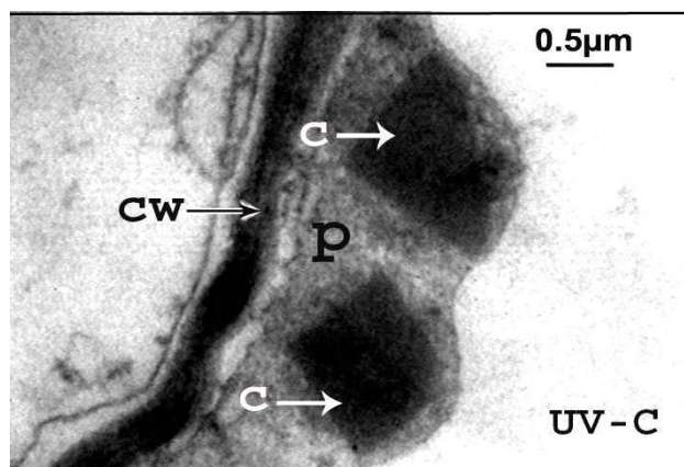
شکل ۱۶. اثر اشعه UV روی تشکیل کریستال‌های پروکسی زومی در سلول‌های مزوفیل گیاهان تیمار در مقایسه با شاهد M، غشای سلولی؛ CW، دیواره سلولی؛ C، کریستال؛ P، پروکسی زوم.
