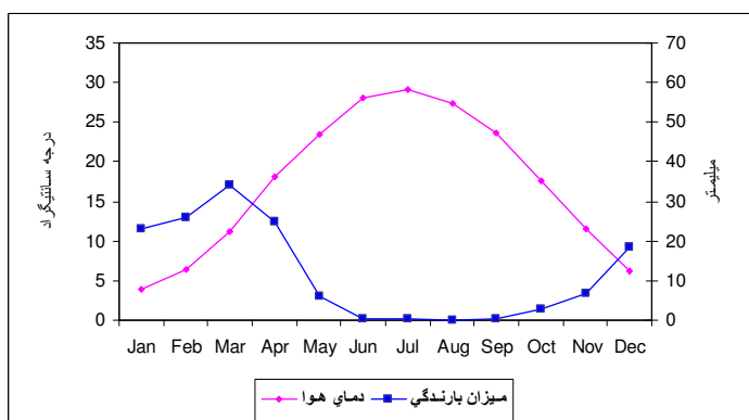
شکل ۱. منحنی آمبروترمیک منطقه بر اساس داده‌های ایستگاه هواشناسی کناباد (۱۹۸۸-۲۰۰۳).
