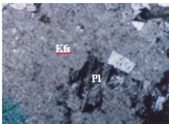
شکل ۵. تصویر بافت پوئی کلینی که در آن فلدسپات پتاسیک پلاژیوکلاز را در بر گرفته است (×100.XPL) فلدسپات پتاسیک = Kfs و پلاژیوکلاز = Pl
