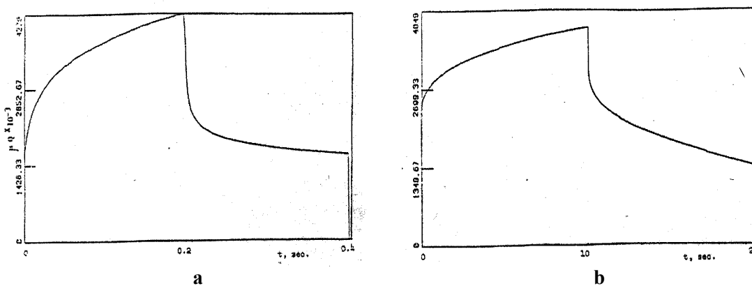
شکل ۴- (a) منحنی کروئوکولومتری الکترودهای نازک طلا 300 \text{ \AA} در الکترولیت 0.1 \text{ M LiClO}_4 ، تغییرات پتانسیل از 0.5 به 0.35 ولت نسبت به SCE (b) منحنی کروئوکولومتری الکترودهای نازک ZnPC ( 1000 \text{ \AA} ) در الکترولیت 0.1 \text{ M LiClO}_4 ، تغییرات پتانسیل از 0.5 به 0.35 ولت نسبت به SCE
