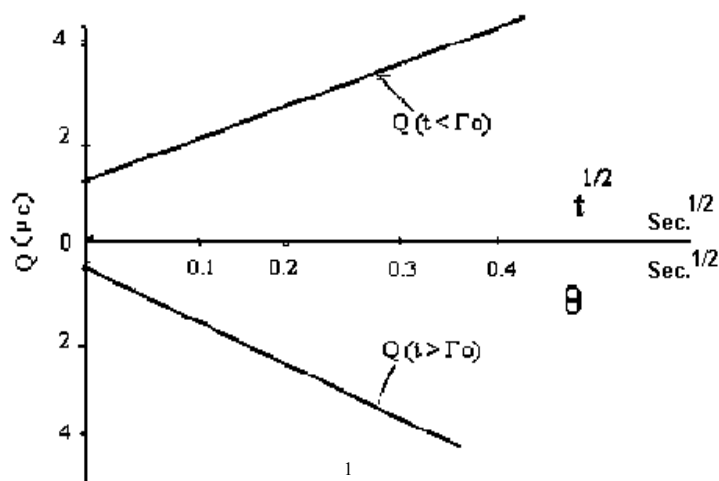
شکل ۳- رسم منحنی Q(t < \tau) نسبت به t^{1/2} و Q(t > \tau) نسبت به \theta
