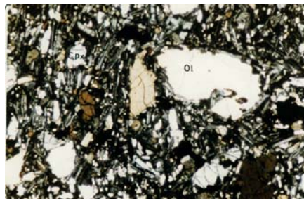
شکل ۱۰ - آلکالی الیوین بازالت با فنوکریستال‌های الیوین و اپاک در زمینه میکروکریستال‌های کلینوپیروکسن پلاژیوکلاز و کانی‌های اپاک (xpl، بزرگنمایی ۲۵x)
