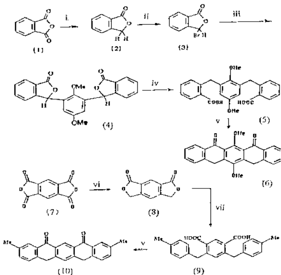
Scheme 1: i, \text{NaBH}_4 ; DMF; ii, NBS, \text{CCl}_4 ; iii, \text{SnCl}_4 ; \text{CH}_2\text{Cl}_2 - P-dimethoxy benzene, iv. \text{Zn} , \text{NaOH} ; v, \text{H}_2\text{SO}_4 or PPA. vi, \text{NaBH}_4 ; DMF; vii, \text{AlCl}_3 ; Toluene.
