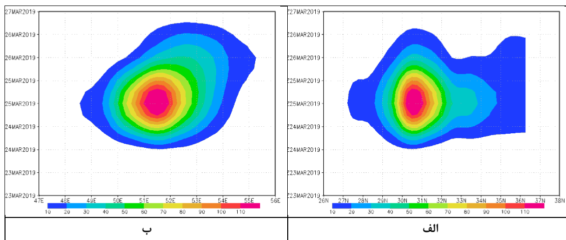
شکل ۱. مقادیر بارش در روزهای ۲۳ تا ۲۷ مارس ۲۰۱۹ در امتداد الف) طول جغرافیایی ۵۱/۵ درجه شرقی و عرض‌های ۲۶ تا ۳۸ درجه شمالی ب) عرض ۳۱/۵ درجه شمالی و طول‌های ۴۷ تا ۵۶ شرقی
