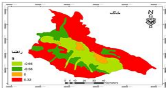
(۶) پهنه‌بندی لغزش بر اساس عامل خاکشناسی
