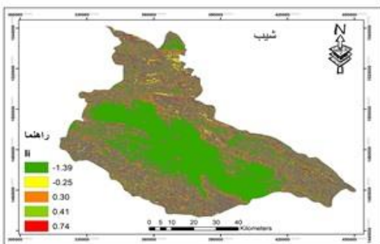
(۴) پهنه‌بندی لغزش بر اساس عامل شیب
