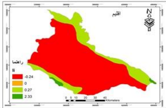
(۳) پهنه‌بندی لغزش بر اساس عامل اقلیم
