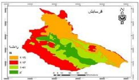
(۸) پهنه‌بندی لغزش بر اساس عامل فرسایش
