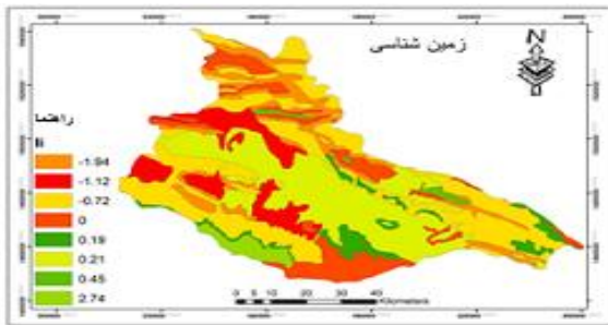
(۵) پهنه‌بندی لغزش بر اساس عامل لیتولوژی
