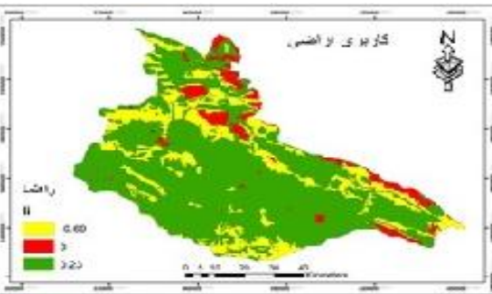
(۷) پهنه‌بندی لغزش بر اساس عامل کاربری اراضی
