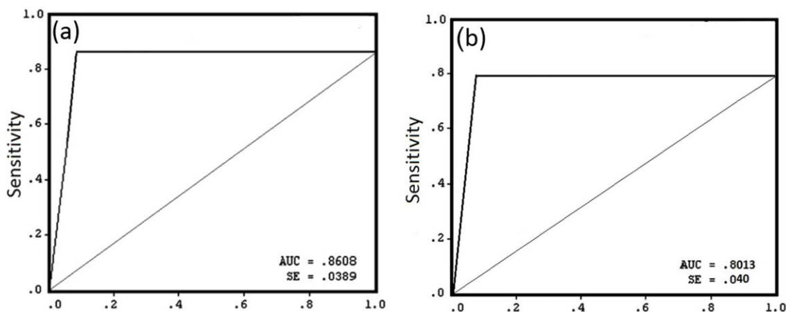
شکل ۷) منحنی ROC مدل شاخص آنتروپی (a) و مدل رگرسیون لجستیک (b)
