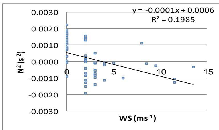
شکل ۵. نمودار پراکندگی پایداری جو ( N^2 ) و تندی باد (WS) در ژانویه سال ۲۰۰۷.
