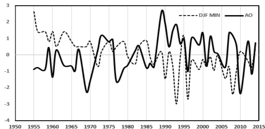
شکل (۷). رابطه و هماهنگی مقادیر استانداردشدهی دماهای حداقل ماهانهی ایستگاه بیرجند در ماههای دسامبر، ژانویه، فوریه، با فازهای منفی و مثبت شاخص AO طی دورهی آماری ۱۹۵۵ تا ۲۰۱۴
