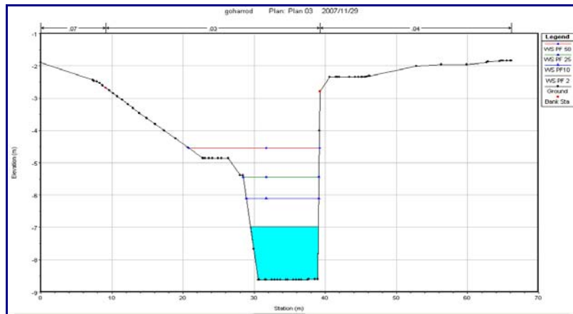
شکل (۸) پروفیل عرضی مقطع شماره ۹۸ رودخانه گوهررود و ارتفاع آب در دوره بازگشتیهای ۲۰، ۲۵ و ۵۰ ساله ( مختصات مقطع در جدول شماره ۲ ارائه شده است)
