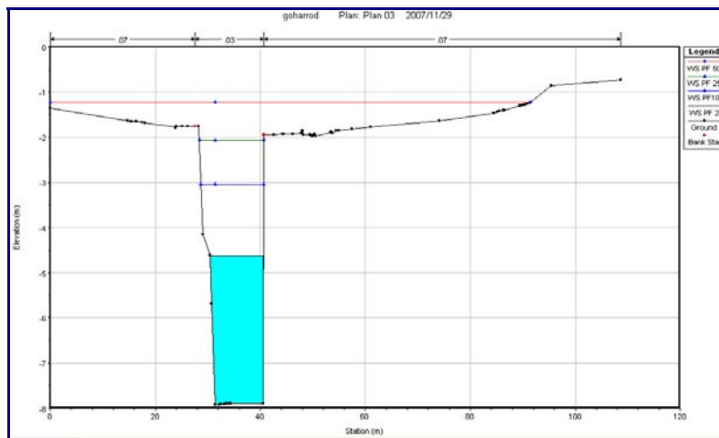
شکل (۹) پروفیل عرضی مقطع شماره ۵۳ رودخانه گوهررود و ارتفاع آب در دوره بازگشتیهای ۲۰، ۲۵ و ۵۰ ساله ( مختصات مقطع در جدول شماره ۲ ارائه شده است)
