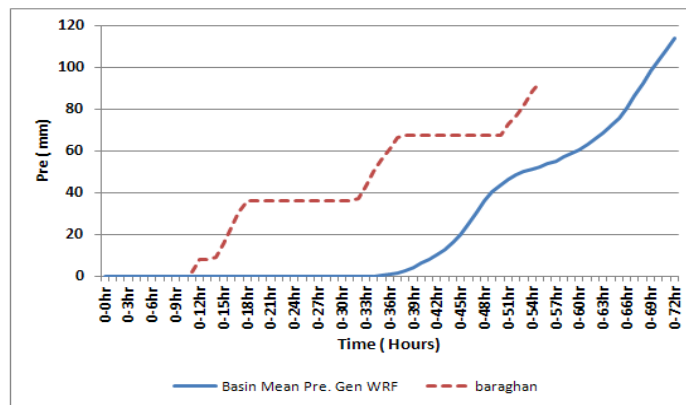
شکل (۴). مقایسه تغییرات الگوی زمانی بارش ایستگاه برغان و مدل عددی WRF (کل حوضه)
