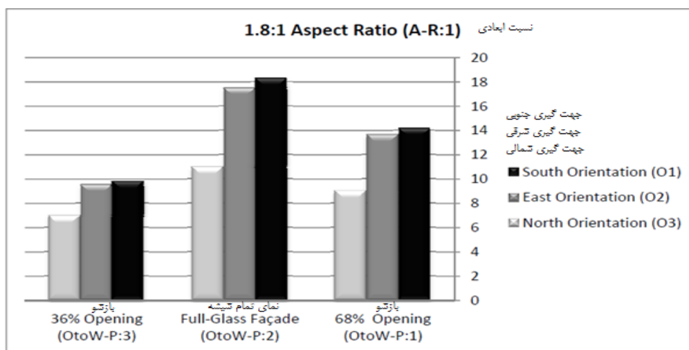
شکل (۳). تاثیر تغییر جهت گیری بر مصرف انرژی سرمایشی در واحدهای نسبت ابعدای 1.8:1 با درصدهای مختلف بازشو به دیوار.
