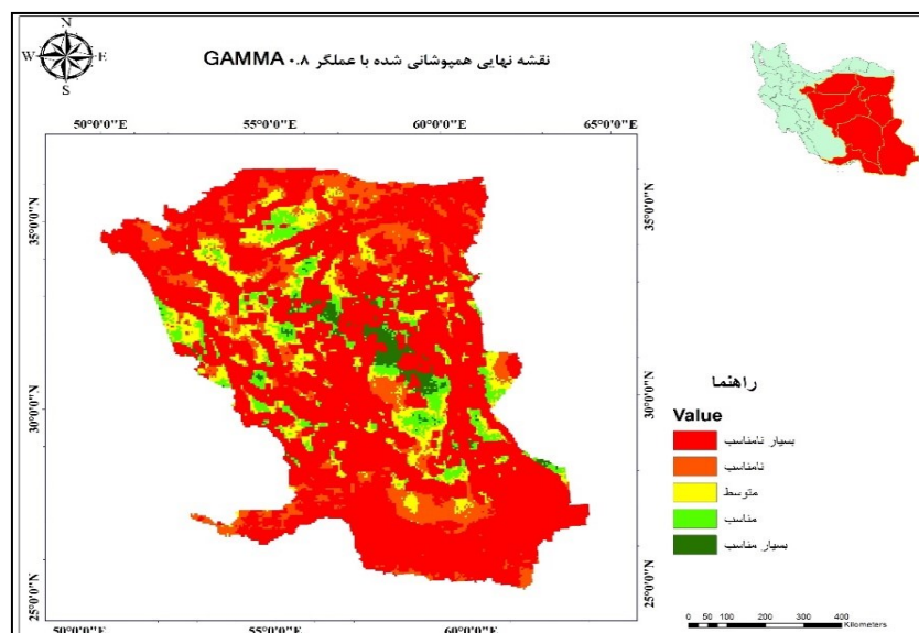
شکل (۷). پهنه‌بندی منطقه از لحاظ کسب انرژی خورشیدی با عملگر 0.8 Gamma
