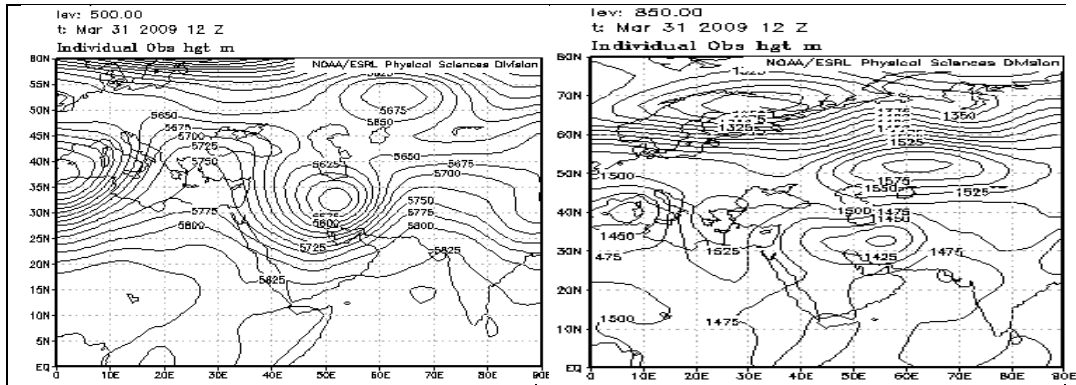
شکل (۷): میدان ارتفاع تراز ۵۰۰ و ۸۵۰ هکتو پاسکال بر حسب متر، ساعت ۱۲:۰۰ گرینویچ روز ۳۱ مارس ۲۰۰۹.
