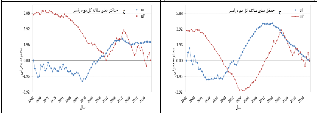
شکل (۲). نمودارهای آزمون ترسیمی من- کندال دمای رامسر
