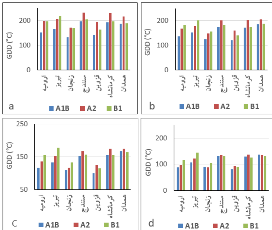
شکل (۴): تغییرات درجه-روز رشد در دوره مطالعاتی ۲۰۱۱-۲۰۲۰ نسبت به دوره پایه بر مبنای آستانه‌های صفر (a)، ۵ (b)، ۱۰ (c) و ۱۵ (d) درجه سانتی‌گراد تحت سه سناریوی مورد مطالعه
