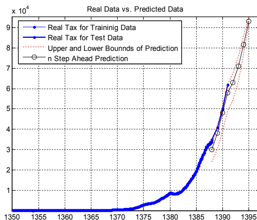
نمودار ۲. پیش‌بینی مالیات بر درآمد برای سالهای ۹۵-۱۳۹۲ با استفاده از الگوریتم PSO
